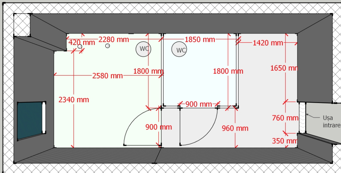
Schița de proiect realizată de Asociația „MOTIVAȚIE” din Moldova, Centru servicii sociale, r. Leova, sat. Cupcui Grupuri sanitare, duș, dimensiuni propuse - 18 iunie 2025 (2/5)
